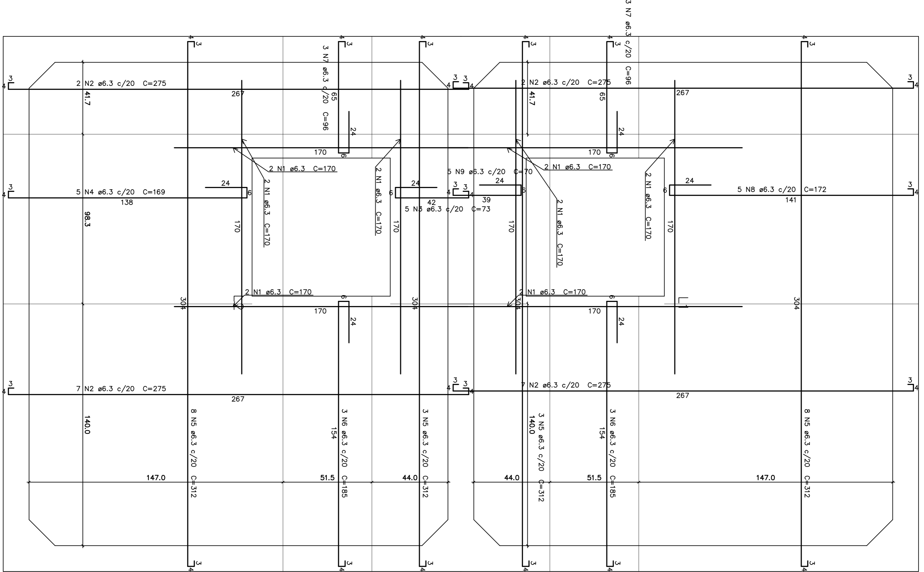
Armação positiva das lajes (10550.0) escala 1:12.5
