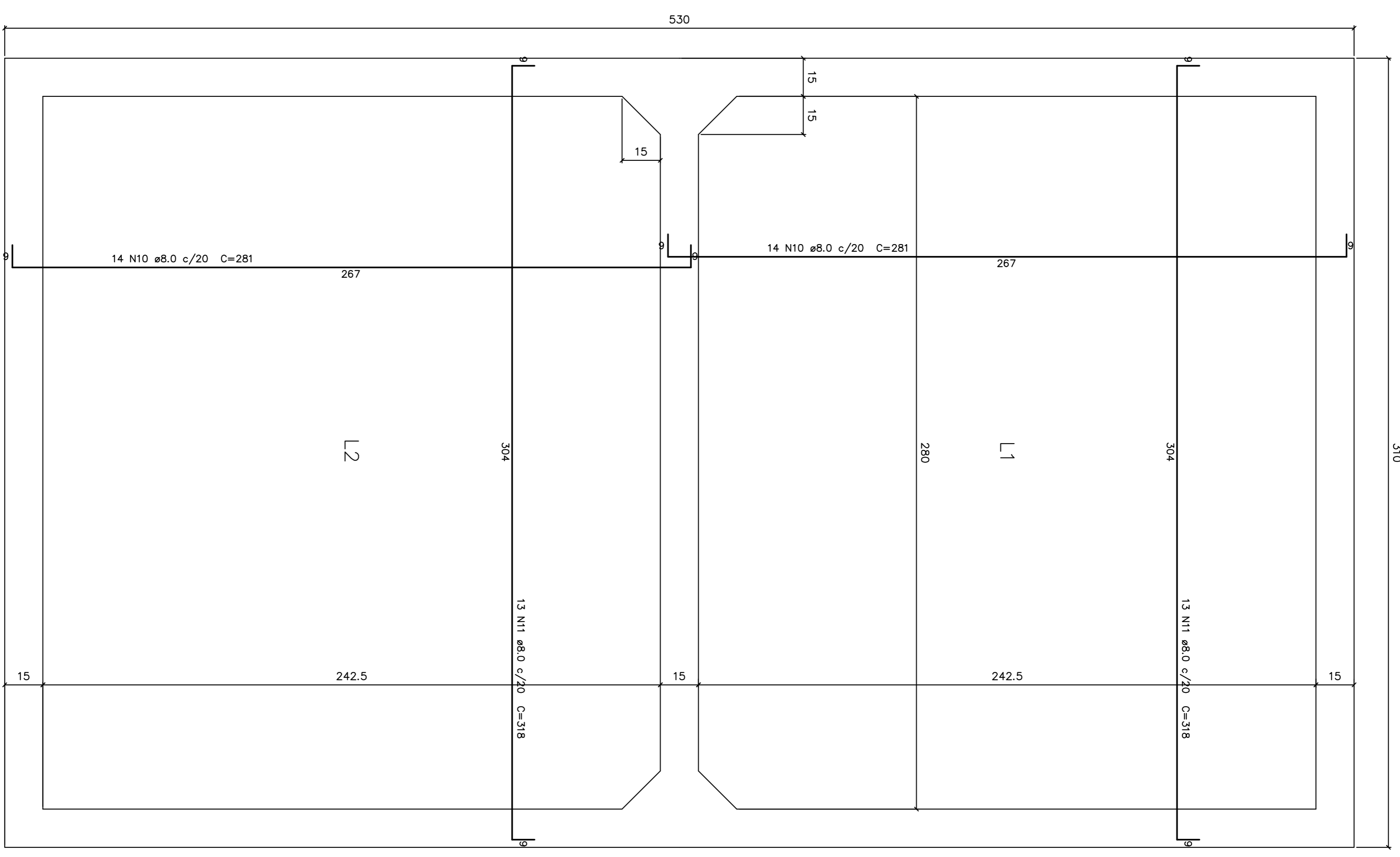
Armação positiva das lajes (10300.0) escala 1:12.5
